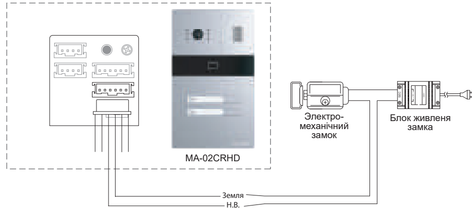
Схема 2. Підключення електромеханічного замка до панелі MA-02CRHD.
