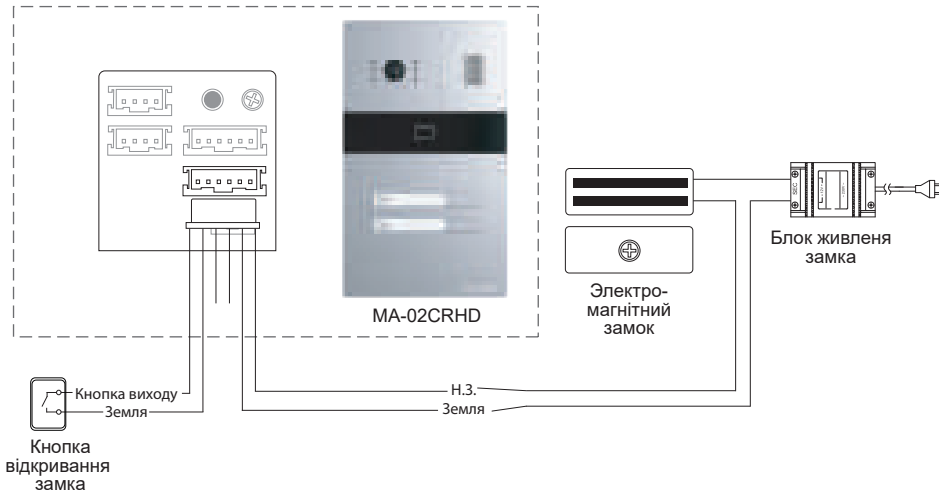
Схема 3. Підключення електромагнітного замка до панелі MA-02CRHD.
