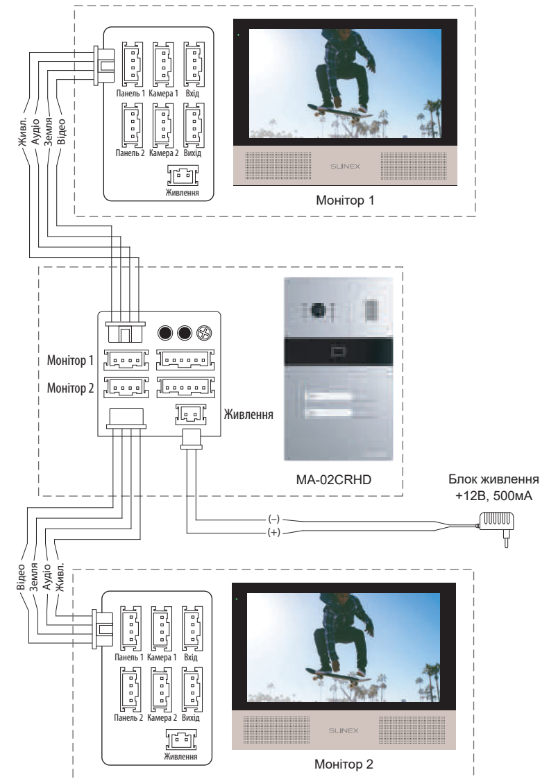
Схема 1. Підключення MA-02CRHD з двома моніторами.
