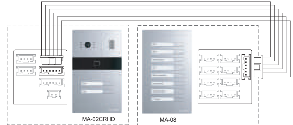
Схема 4. Підключення MA-02CRHD та MA-08.
