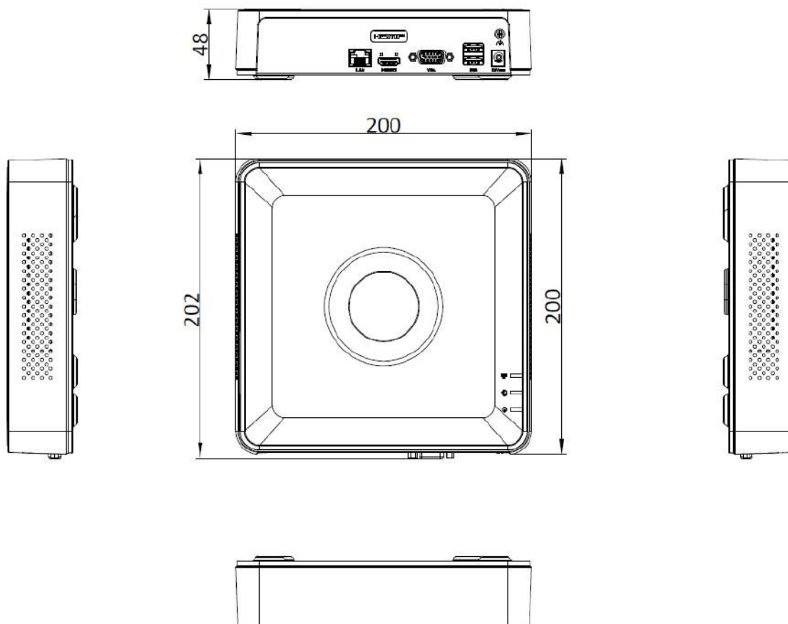
scale/1:1;Unit/mm
